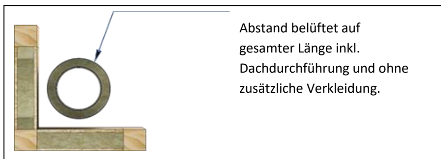
Abbildung 2: Abstand zu brennbaren Materialien
